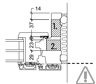
VELFAC In, 123mm frame 1. + 2. ⇒ see text
