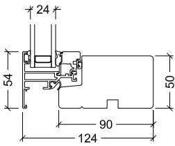
VELFAC 200 DGU
